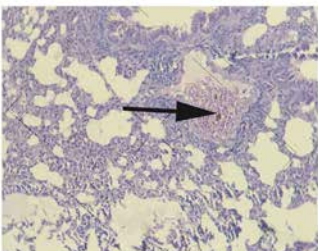
Metastasis + Curculigoside
